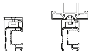
Distanzplatte für zweite Führungsschienseite bei Montage mit Seitenbefestigung oder Montageverlängerung
